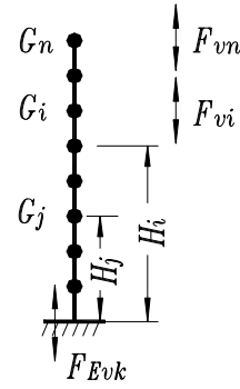
图4.3.2 结构竖向地震作用计算简图
